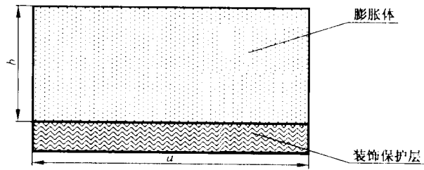
图 1 复合膨胀体典型结构型式
